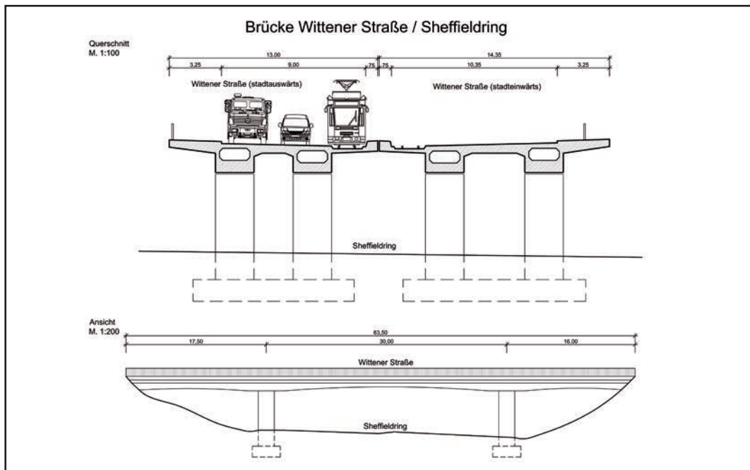
Der Quer- und Längsschnitt zeigt den Aufbau der Spannbeton-Brücke.
